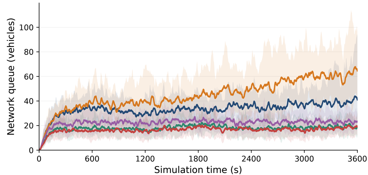
PPO
