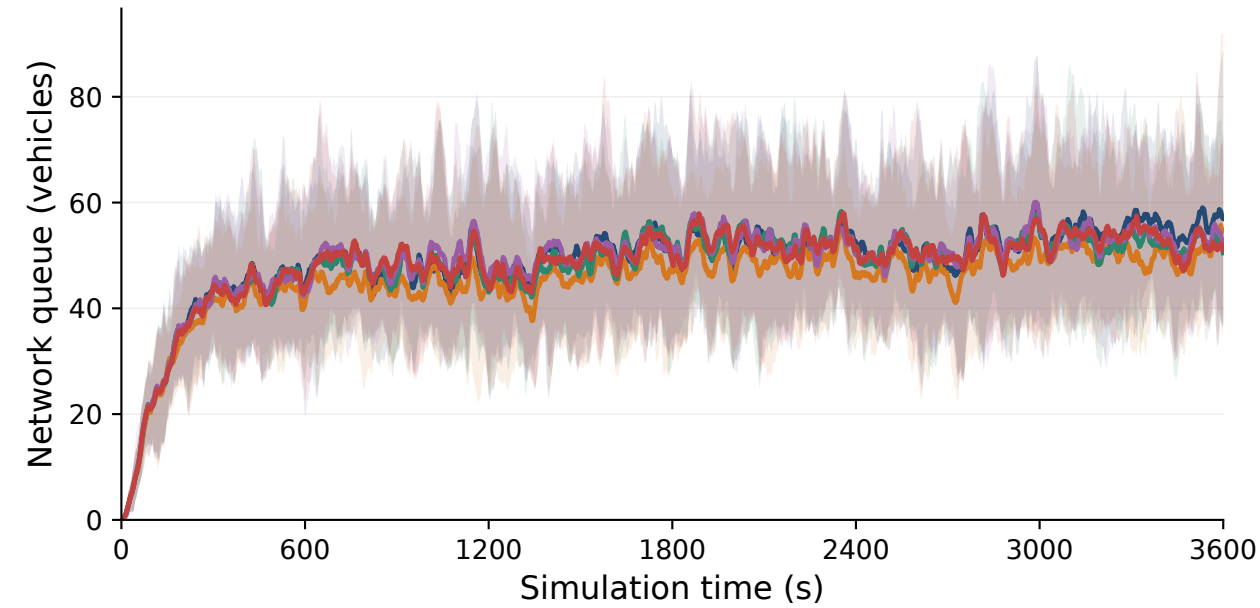
MA2C
