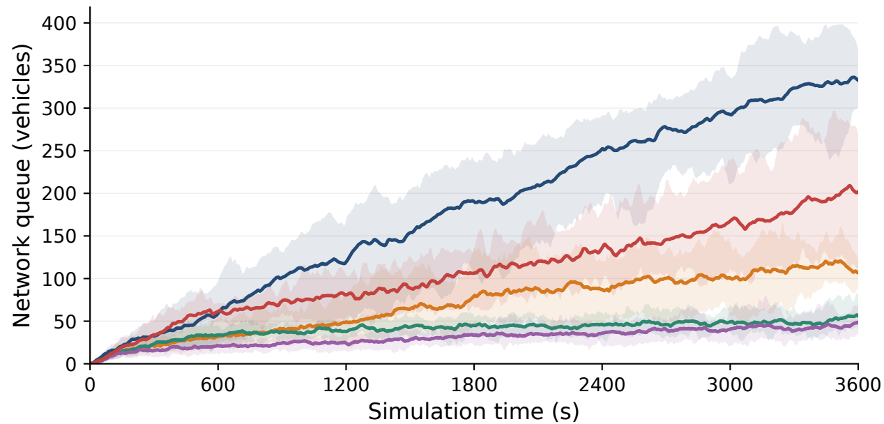
IQLL
